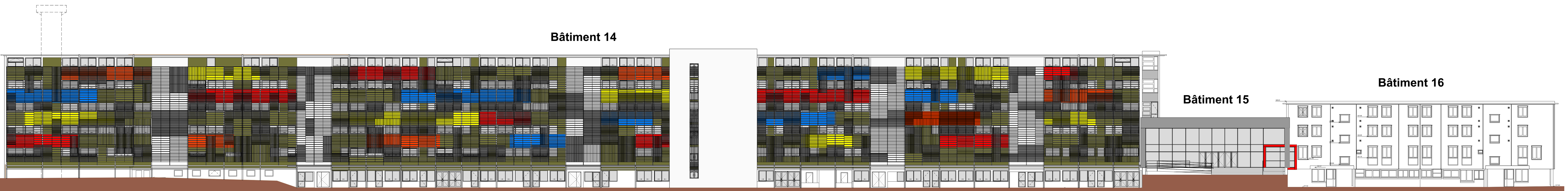
ELEVATION NORD - AVEC RÉSILLE
