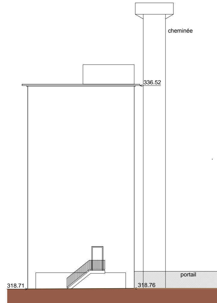
Elévation Est - Bâtiment 14
